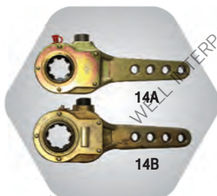
14A ขาปรับเบรก 8 ฟัน 4 รู ร่องฟัน 38 mm 14B ขาปรับเบรก 8 ฟัน 4 รู ร่องฟัน 42 mm
