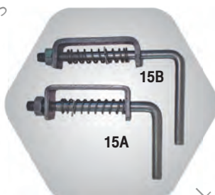
15A ขอล็อคฝาท้าย 5/8" 15B ขอล็อคฝาท้าย 3/4" พร้อมสปริง
