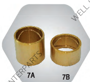
7A บัชทองเหลืองโดงแดง CIMC 60x68x62 mm 7B บัชทองเหลืองเต้าโดงแดง CIMC 60x70x40 mm
