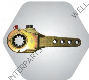
7 ขาปรับเบรก 10 ฟัน 4 รู
