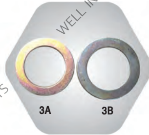
3A แหวนรอง MAG สี่ทอง 57x39x1.5 mm 10-3500A 3B แหวนรองแกนลูกเบี้ยว YORK 500358
