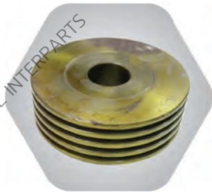
6A ลูกสูบดัม 183 mm 4 ร่อง (มีรู 40 mm/50 mm)
