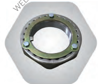
12 ชุดแหวนล็อกปรับหัวเพลลา MAGNUM แบบหนา
