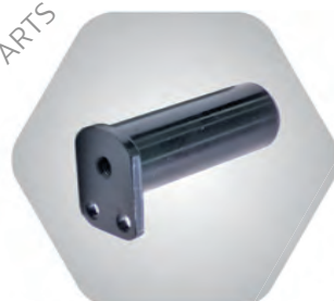
15 สลักฐานจานลาก PCM K, JOST 36
