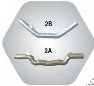
2A สปริงพืน MAGMUN I 2B สปริงพืน MAGMUN II, ROR, YORK
