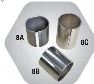
8A บัชแองเคอร์พิน Fuwa/Fuhe 8B บัชแองเคอร์พิน MAGNUM II, ROR, YORK 8C บัชแองเคอร์พิน MAGNUM I
