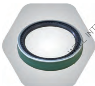
14 ซีลเพลลา YORK เขียว 117.5-152.3-25.5 #786114-B318
