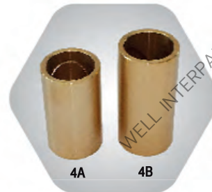
4A บัชทองเหลืองโดงแดง 3" 62x50x105 mm 4B บัชทองเหลืองโดงแดง 4" 62x50x125 mm
