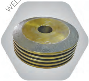
9A ลูกสูบดัม 220 mm 3 ร่อง รู 50 mm 9B ลูกสูบดัม 220 mm 4 ร่อง รู 45 mm 9C ลูกสูบดัม 225 mm 4 ร่อง รู 50 mm
