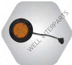
1 โฟลติดูปแลมปกลม 2.5" LED SOS สีเหลือง (มี 24Vdc/9-33Vdc)
