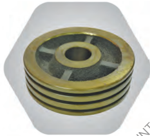
2 ลูกสูบดัม 170 mm รู 40 mm (มี 3 ร่อง/4 ร่อง)
