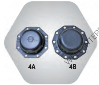
4A ฝาครอบคัม ZM 8 รุ 4B ฝาครอบคัม ZM 10 รุ
