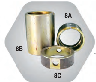
8A บัชก่ายลัดม SMM 60x72x50 mm 8B บัชก่ายลัดม SMM 60x75x104 mm 8C แหวนลัดมเพลาก่ายลัดม SMM 60x75x22 mm
