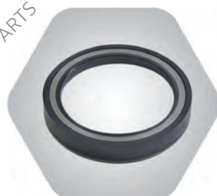
15 ซีลเพลลา YORK ขอบยาง 117.5-152.3-25.5 #B370025-BG204226
