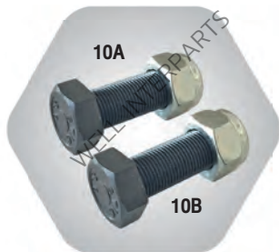
10A ชุดสกรูยึดจานหมุน M16x50 (เกลียวละเอียด) 10B ชุดสกรูยึดจานหมุน M18x50 (เกลียวละเอียด)
