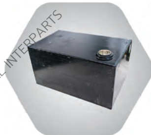
6 ถังน้ำมันไฮดรอลิคเหลี่ยมเล็ก 43L
