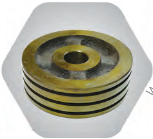
5A ลูกสูบดัม 180 mm 3 ร่อง รู 50 mm
