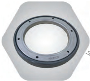
5A ซีลเพลลา Fuwa #376590X 5B ซีลเพลลา Fuhe 1301WF 108-152.3-17.5
