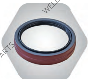
13 ซีลเพลลา YORK แดง 117.5-152.3-25.5 #B370025BG
